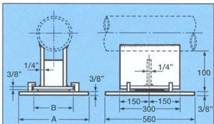
PARA TUBOS DE DN 8" ATÉ DN 12"
