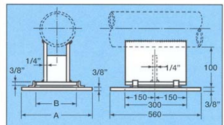
PARA TUBOS DE DN 8" ATÉ DN 12"
