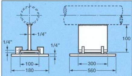
PARA TUBOS DE DN 2" ATÉ DN 6"
