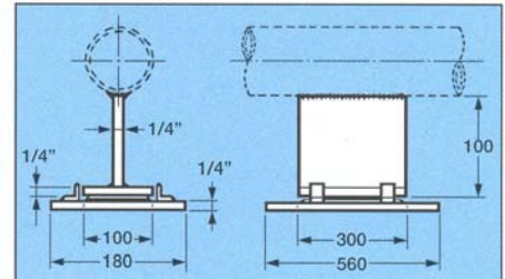
PARA TUBOS DE DN 2" ATÉ DN 6"
